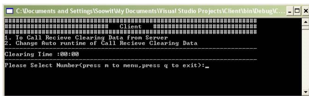
รูปที่4-27 ส่วน Software Engine ซึ่งทำหน้าที่ไปขอเซอร์วิส ข้อมูลการจ่ายเงิน(Clearing)
